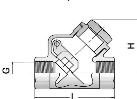
šikmé provedení
