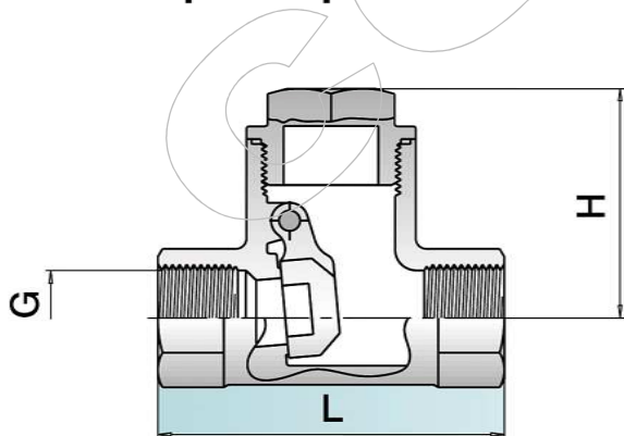
přímé provedení
