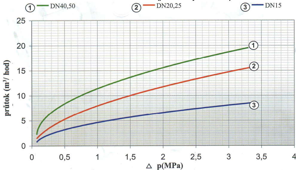
Průtoková charakteristika KOMO 4 DUO (pro studený kondenzát)
