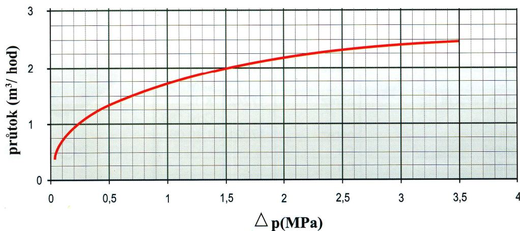
Průtoková charakteristika KOMO 4 midi (pro studený kondenzát)
