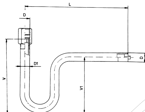
smyčka zahnutá s čepem AN 137530 DRUH A
