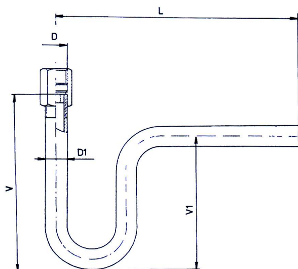
smyčka zahnutá přivařovací AN 137530 DRUH B
