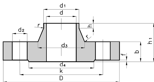
d 4 hladká těsnící lišta
