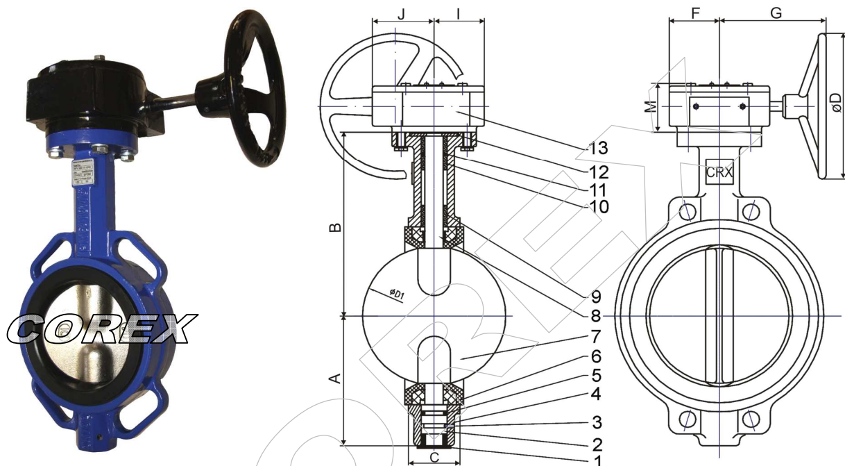
Rozměry převodovky / Gearbox data
