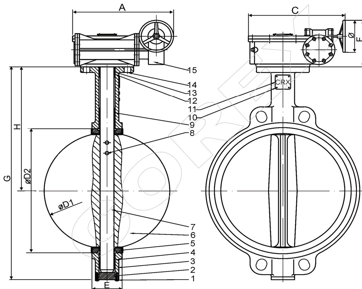
Tabulka rozměrů / Table of dimensions
