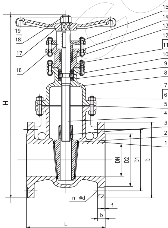
Tabulka rozměrů (mm) / Table of dimensions (mm)
