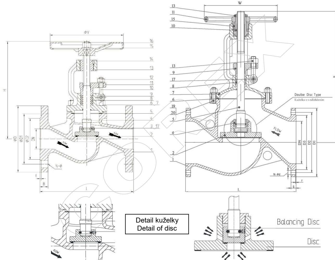
Tabulka materiálů / Materials specification DN65 - DN150
