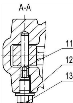
Detail závěsu talíře Detail of hinge pin
