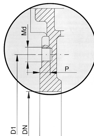
detail slepého otvoru
