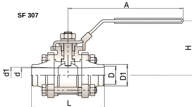
Tabulka rozměrů :
