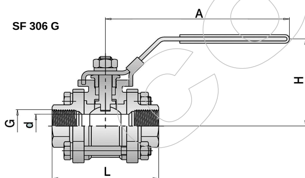
Tabulka rozměrů :
