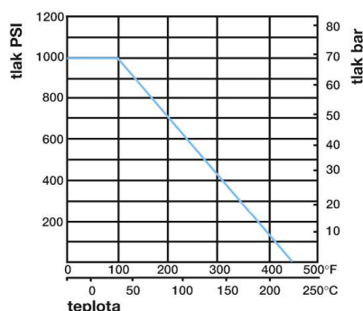
diagram závislosti tlaku na teplotě
