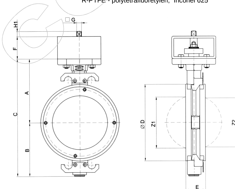
Tabulka rozměrů
