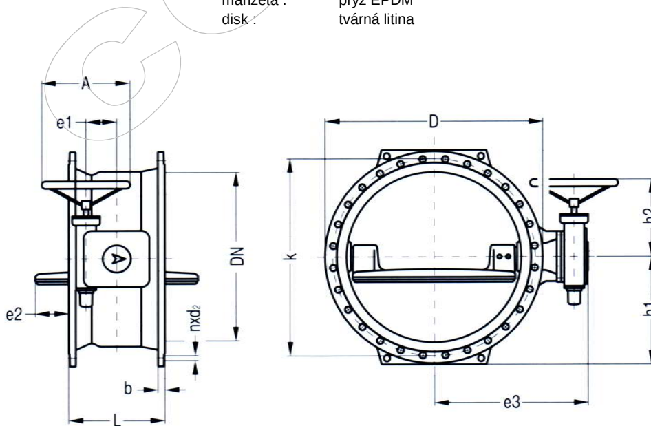
Tabulka rozměrů pro provedení PN 10 pozn. (pro PN6, 16, 25 a DN 1600 a 1800 si vyžádejte katalogový list v naší firmě)
